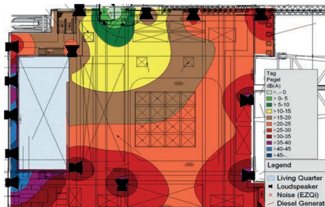
Abb. 5: Darstellung des Signal-Rausch-Abstands
