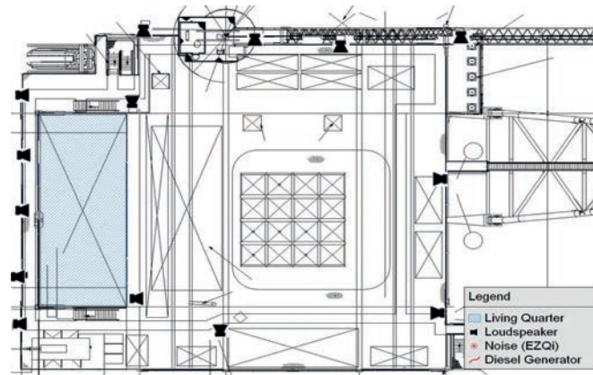
Abb. 2: Lautsprecherübersichtsplan
