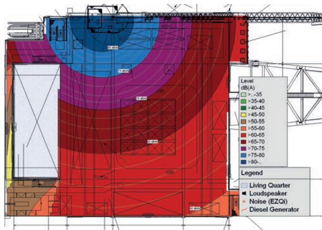
Abb. 1: Darstellung der Umgebungsgeräusche
