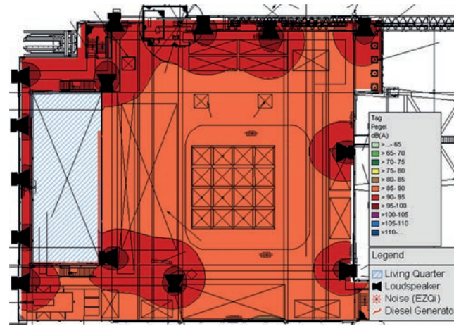
Abb. 3: Abstrahlverhalten der Lautsprecher
